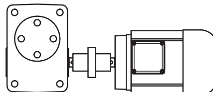
Martinetto con albero di entrata giunto motore con fissaggio a piedi
